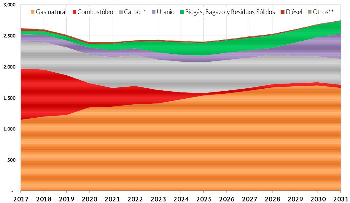
GRÁFICO 4.6.1. CONSUMO DE COMBUSTIBLES 2017-2031
