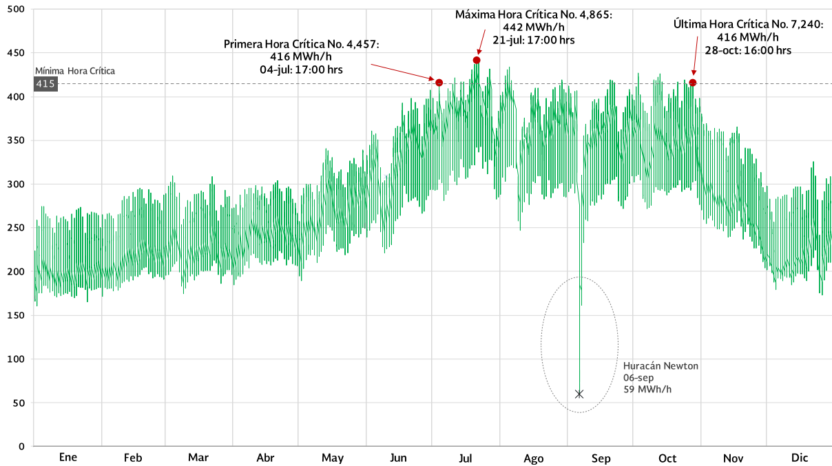
GRÁFICO 3.3.5. CURVA DE DEMANDA HORARIA DE BAJA CALIFORNIA SUR 1/ 2016 (Megawatt-hora/hora)
