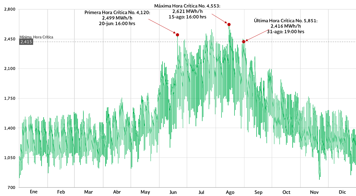
GRÁFICO 3.3.3. CURVA DE DEMANDA HORARIA DE BAJA CALIFORNIA 2016 (Megawatt-hora/hora)
