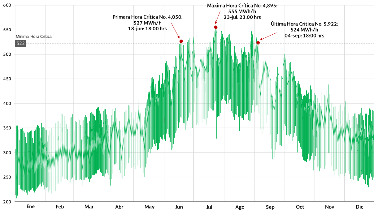
GRÁFICO 3.3.6. CURVA DE DEMANDA HORARIA DE BAJA CALIFORNIA SUR 1/ 2022 (Megawatt-hora/hora)
