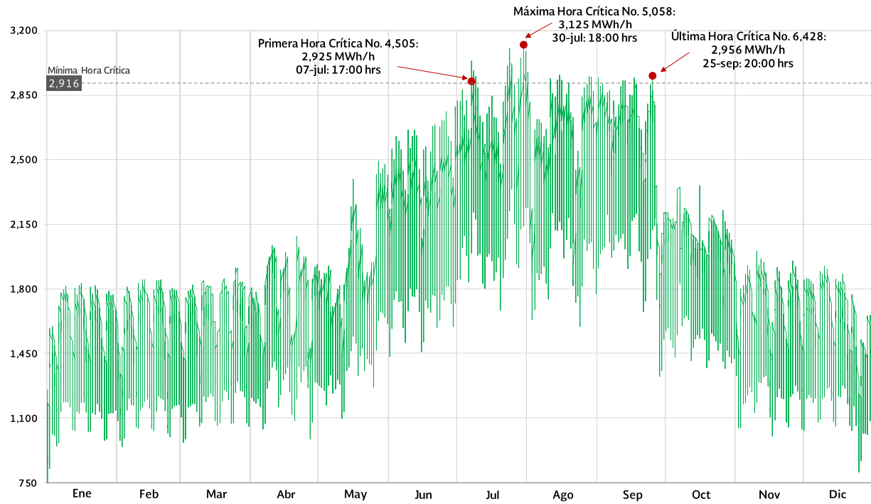
GRÁFICO 3.3.4. CURVA DE DEMANDA HORARIA DE BAJA CALIFORNIA 2022 (Megawatt-hora/hora)
