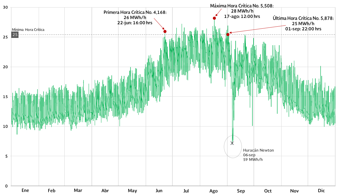
GRÁFICO 3.3.7. CURVA DE DEMANDA HORARIA DE MULEGÉ 2016 (Megawatt-hora/hora)
