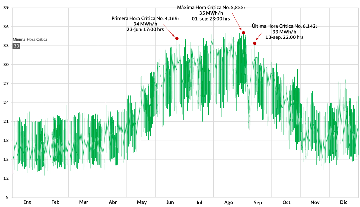
GRÁFICO 3.3.8. CURVA DE DEMANDA HORARIA DE MULEGÉ 2022 (Megawatt-hora/hora)
